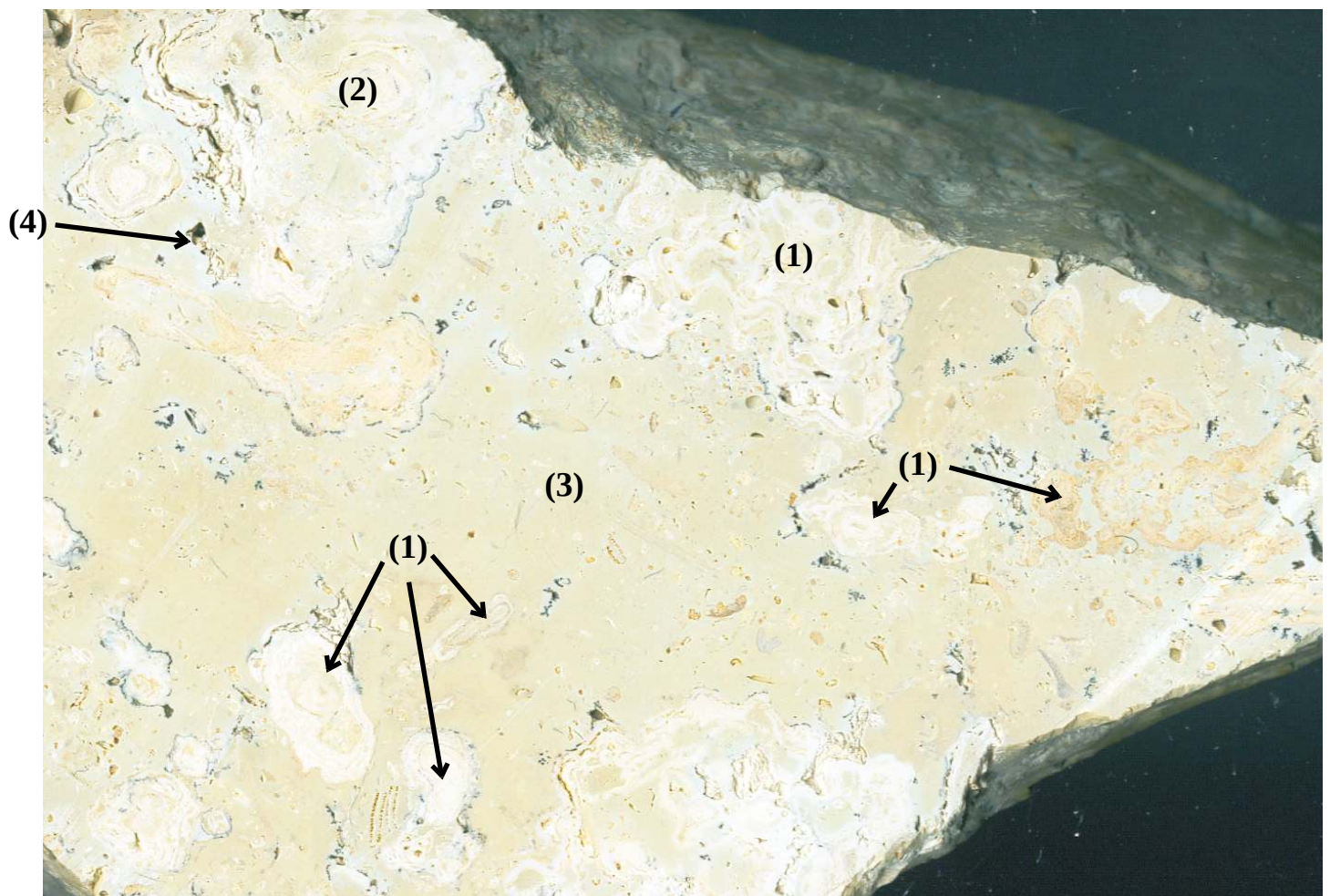
108_2 : Calcaire lacustre à algues (x 2.5), surface polie
